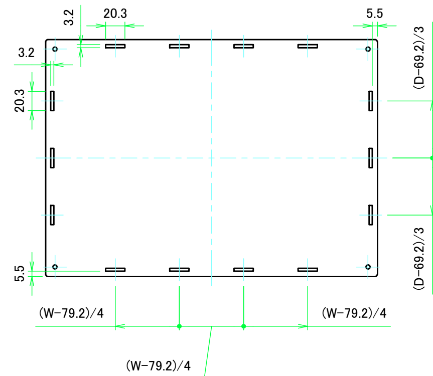
上カバー裏面 / Top cover Backside
